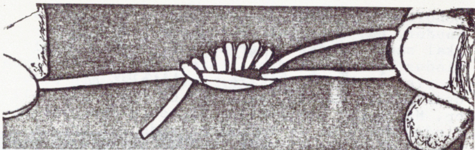
Øjeløkke på lineenden (forfangsløkke). Denne knude bindes med linen lagt dobbelt.
